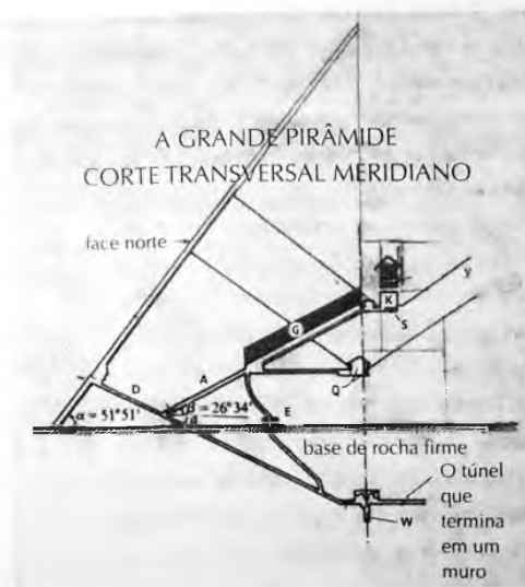
Ilustração 9-41. Corte transversal da Grande Pirâmide.
